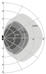
Patrón de montaje de detección (Unidad: m) Altura de instalación sugerida: 1-1.8 m
