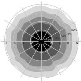
Patrón de montaje de techo (Unidad: m) Altura de instalación sugerida: 2.5-8m
