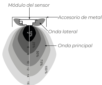
Patrón de montaje de detección (Unidad: m) Altura de instalación sugerida: 1-1.8 m
