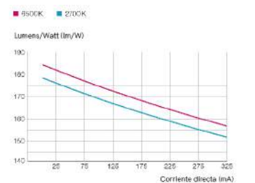
Eficacia en función de la corriente directa
