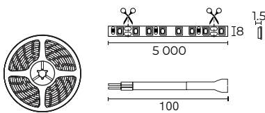
CORTE CADA 50 mm / 6 LEDs
