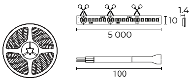
CORTE CADA 33.3 mm / 7 LEDs
