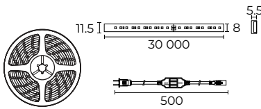
CORTE CADA 500 MM / 60 LEDs
